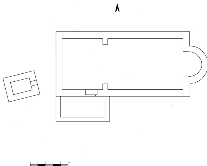
Сл. 3. Ситуациони план
